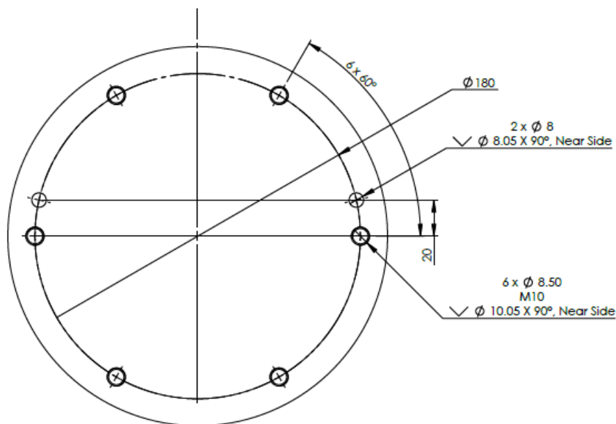
1.1: Ansicht der Roboterbasis von unten
